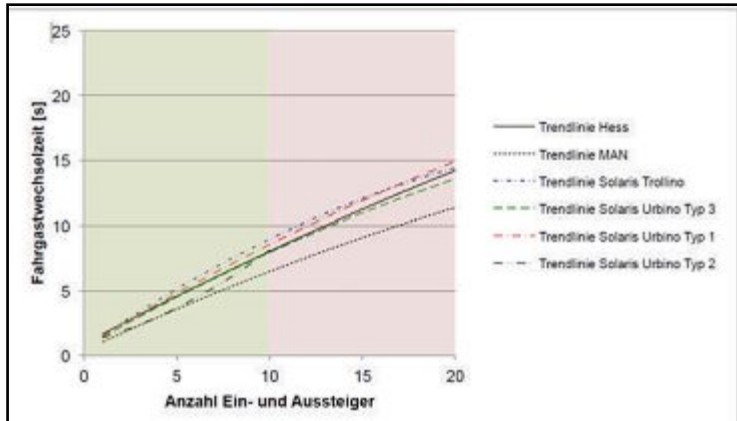
Fahrgastwechsel vs. Fahrplanwechselzeit, Bsp. Haltest. «Stadthaus, stadteinwärts»
